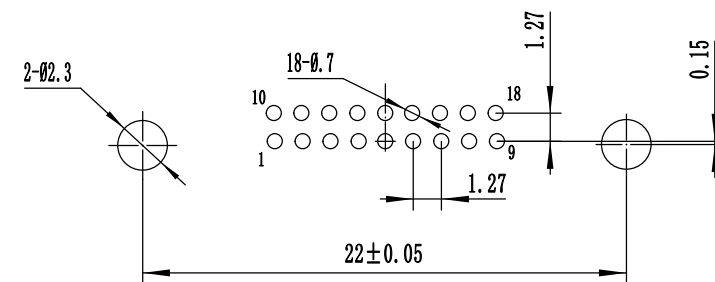
PCB开孔尺寸图
