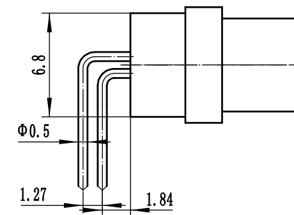
侧面 (去除附件)
