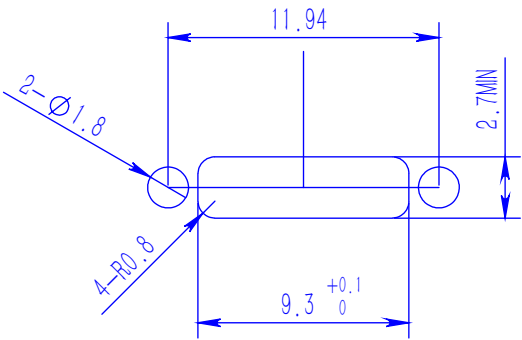
安装开孔尺寸 (出线端)
