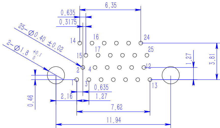
印制板开孔推荐图 (插装面)
