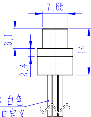
去附件视图
