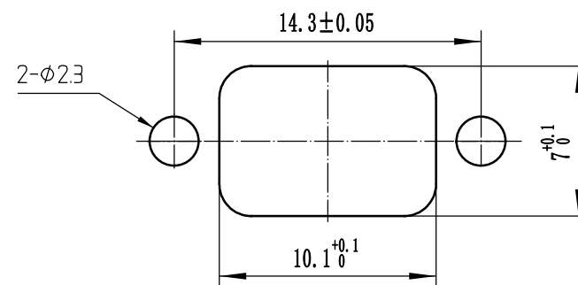
面板开孔尺寸 (板前安装)
