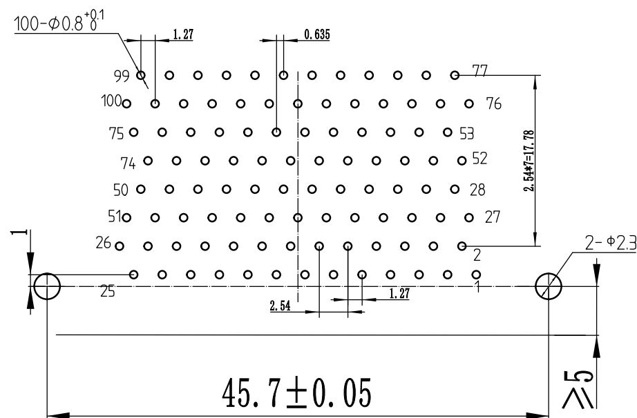
PCB开孔尺寸图
